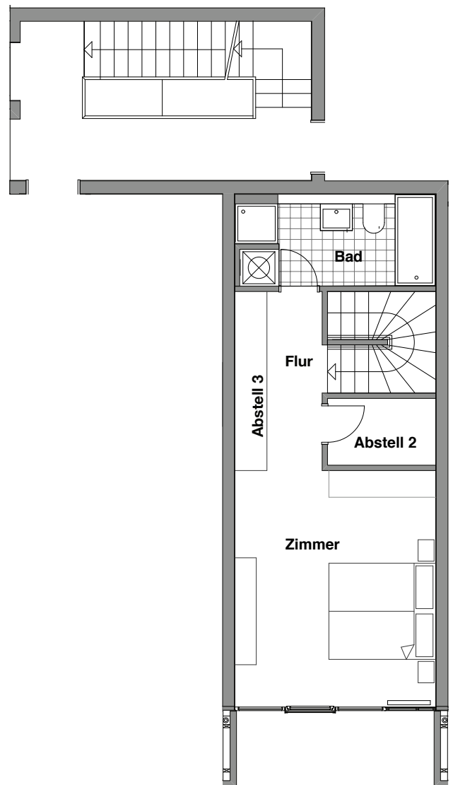
2. Obergeschoss
